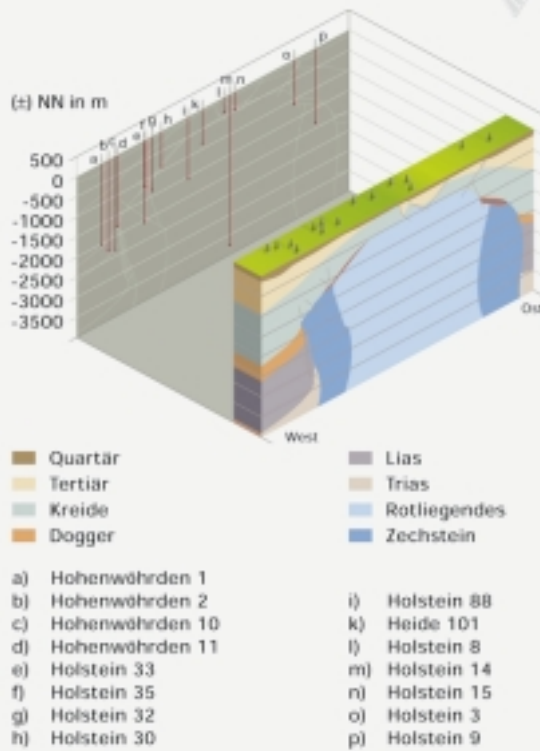
Querschnitt durch den Salzstock Heide
